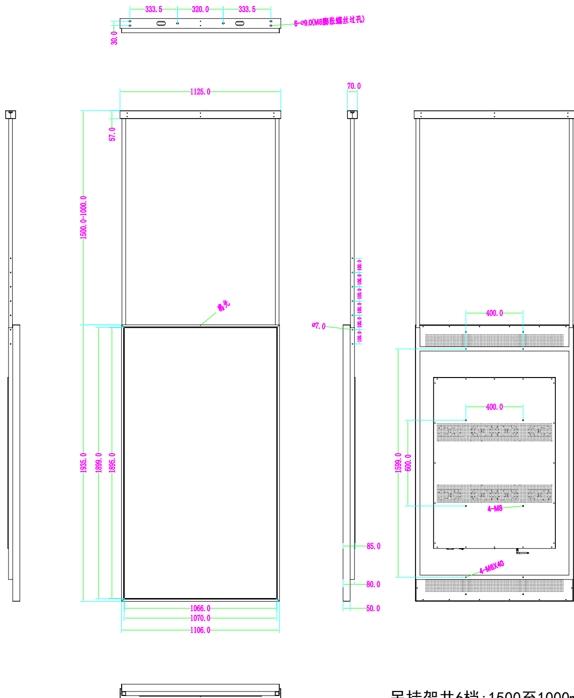
吊挂架共6档: 1500至1000mm
