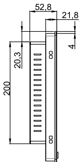
前置USB12.1寸外嵌式（散热款）
