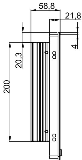
前置USB12.1寸外嵌式（全封闭）
