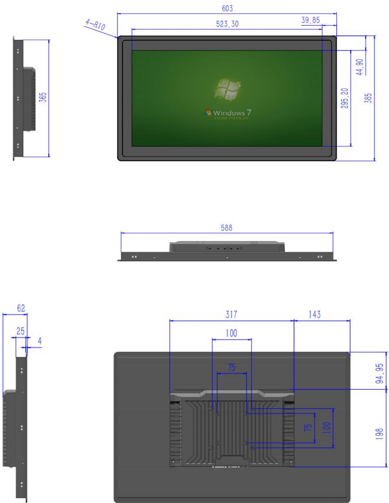
产品尺寸图（23.6 寸全封闭防尘显示器）
